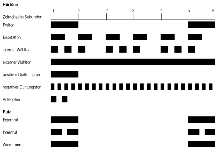
Höröne und Rufakte von Eumex 2220PC am angeschlossenen Telefon
