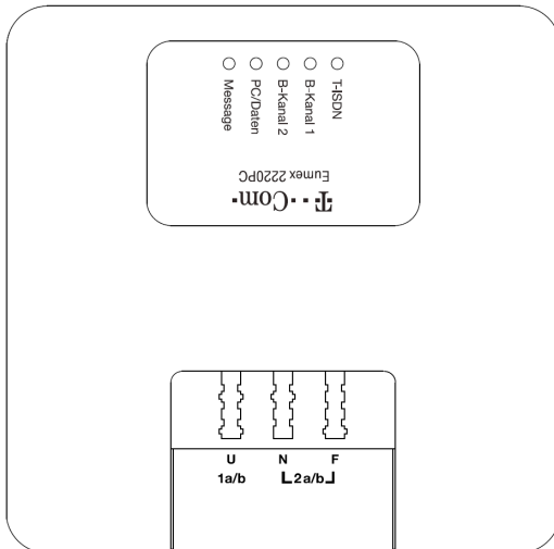
TAE-Buchsen und Leuchtdioden – Draufsicht von Eumex 2220PC
